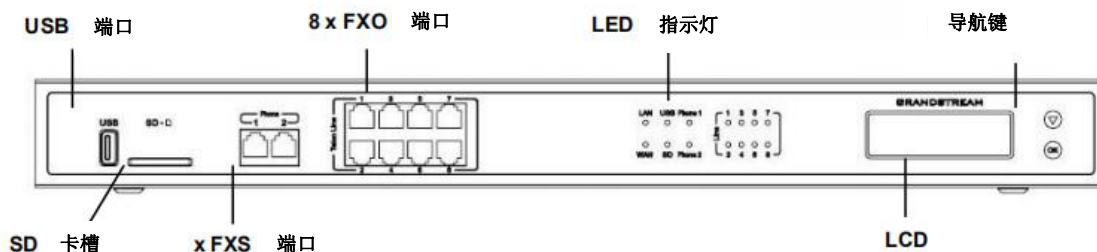
图 5: UCM6208 正面图
