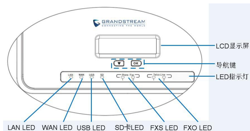
图 2: UCM6202 背面图
