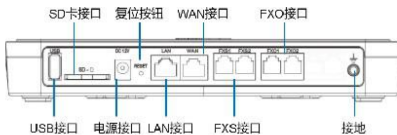
图 1: UCM6202 正面图
